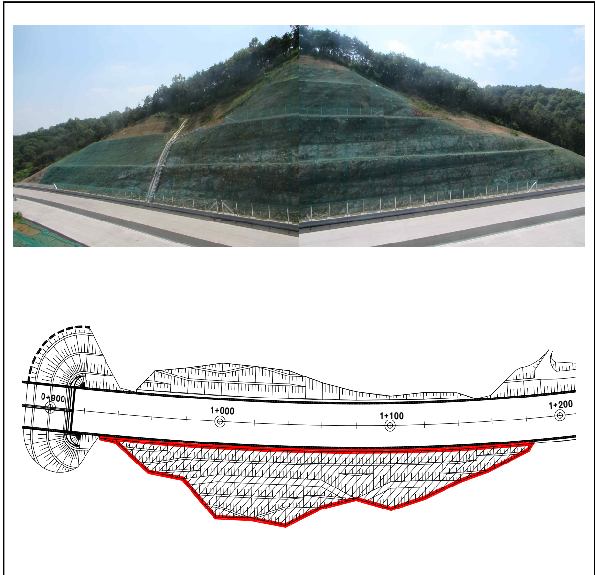
【그림 28.14】 영천절토28 검토대상 비탈면구간
